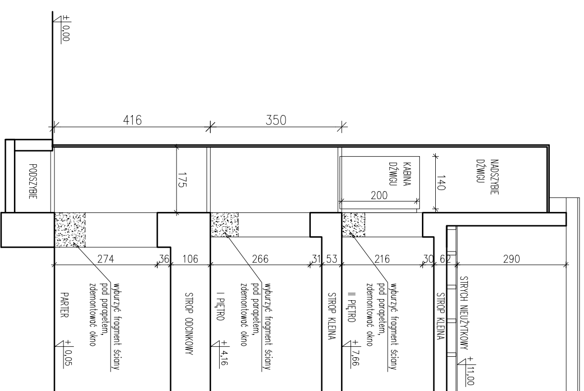
PRZEKRÓJ B-B/ PROJEKTOWANY DZWIĘG OSOBOWY
